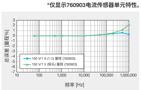
零功率因数下的频率—功率精度特性
